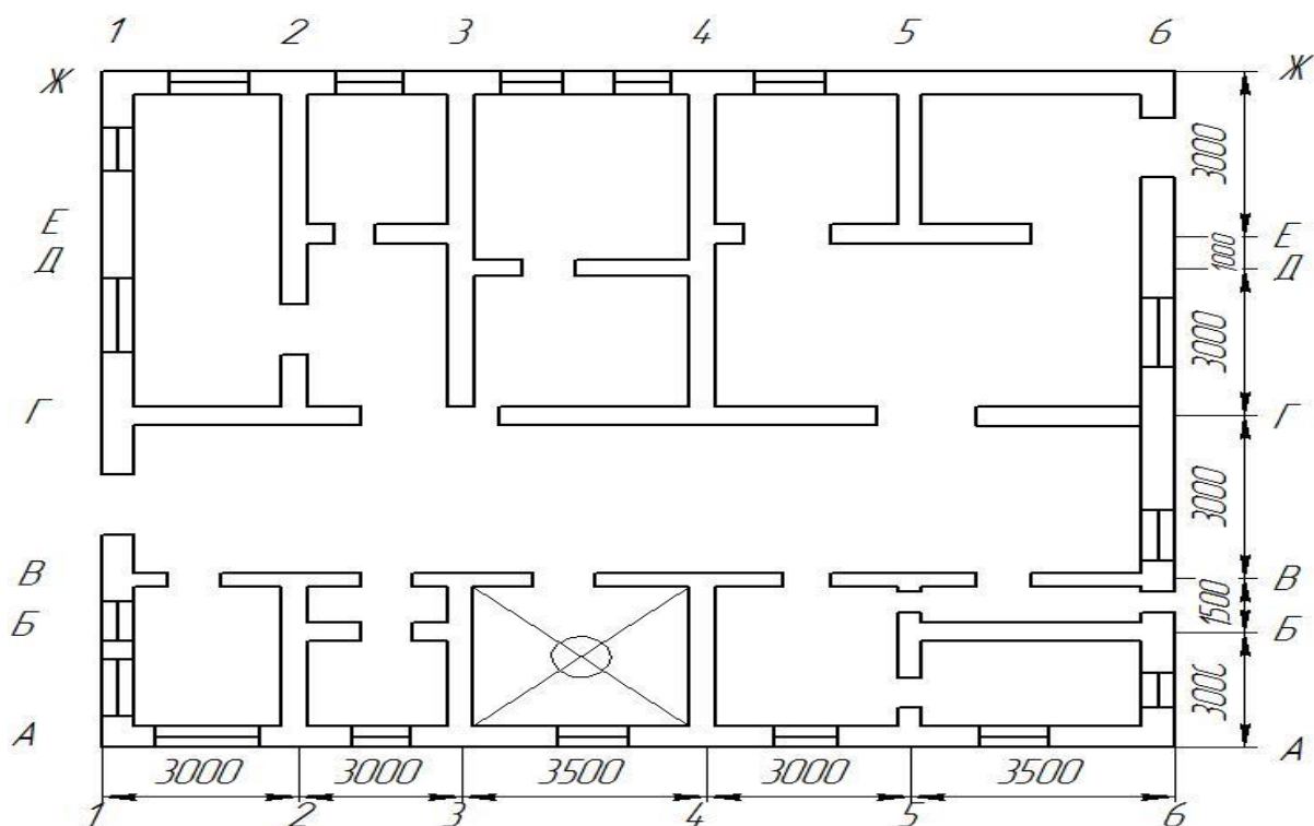
Рисунок 1 - План здания
